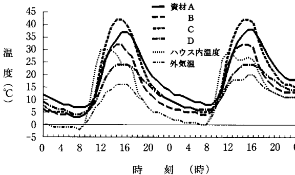
第1図 被覆資材別の床土温度の推移 (1992年2月26～27日)
